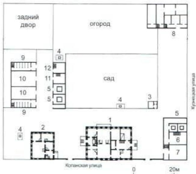
План усадьбы В. Б. Хохрякова. Обмер 1816 г.
