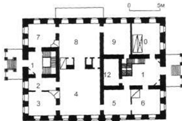
План первого этажа дома В. Б. Хохрякова. Обмер 1816 г.
